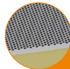
Foratura R4T6 • Rapporto vuoto/pieno 42% R4T6 Drilling • Solid/void ratio 42%
